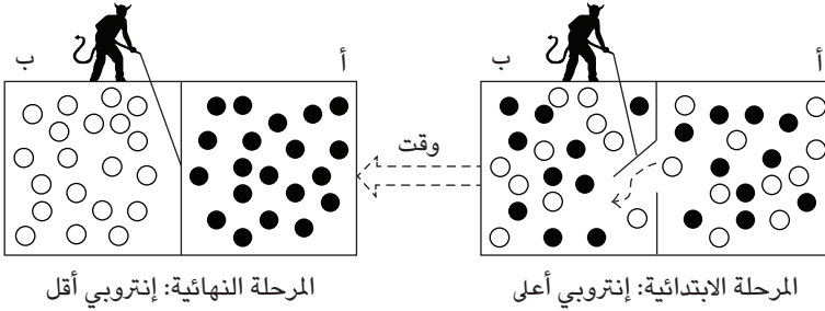
شكل ٥-٢: شيطان ماكسويل.
