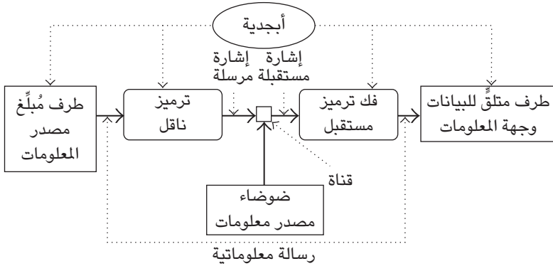
شكل ٢-٣: نموذج اتصال.
